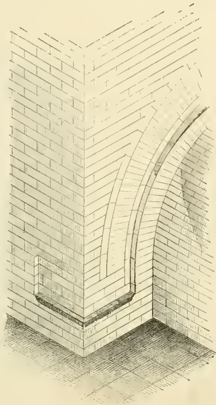
91. — Retour d'angle de l'archivolte d'une porte de la ville. D'après le géométral de Place, t. III, pl. 48.
